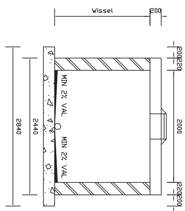
SNIT B-B
