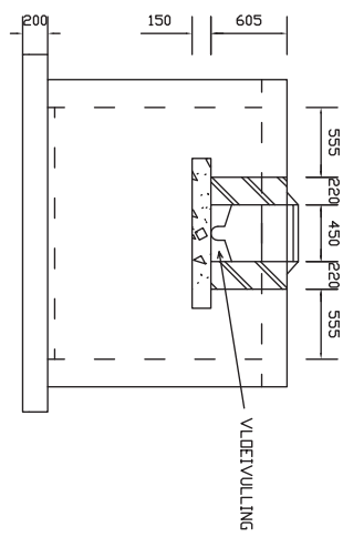
SNIT C-C
